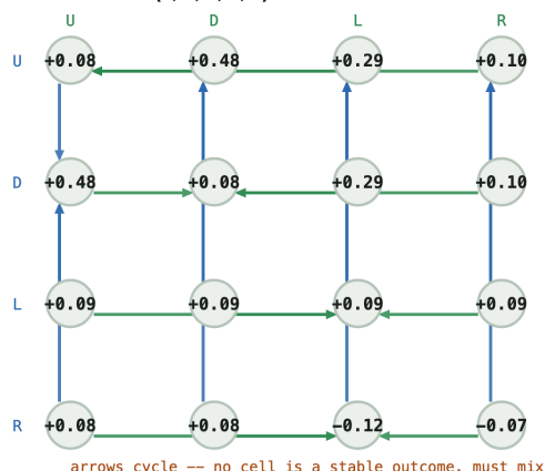
Q matrix -- (0, 2, 1, 2, 0)
