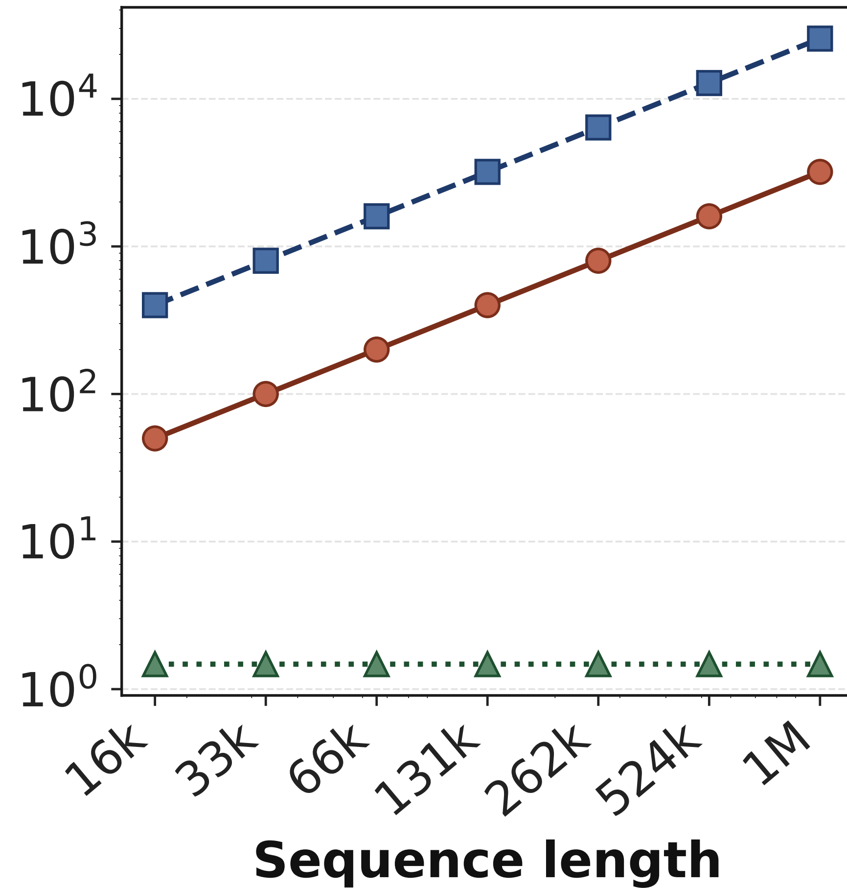
KV Cache (GB)
