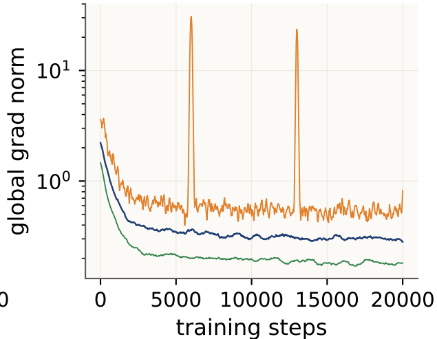
Gradient norm
