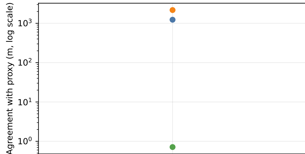
APE RMSE
