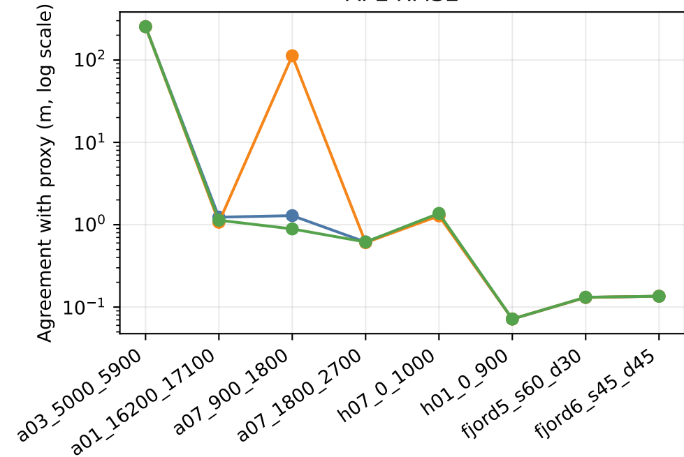
APE RMSE
