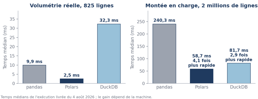
Temps médians de l'exécution livrée du 4 août 2026 ; le gain dépend de la machine. Figure 2. Temps médian des trois moteurs au volume réel, puis sur deux millions de lignes (exécution livrée du 4 août 2026). Figure redessinée à partir des sorties du notebook (mêmes données).
