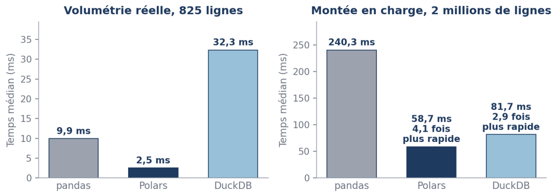
Figure 1. Temps médian des trois moteurs, au volume réel puis sur deux millions de lignes (exécution livrée du 4 août 2026). Figure redessinée à partir des sorties du notebook (mêmes données).
