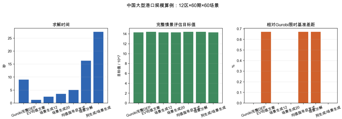
图 4: 真实港口规模算例下不同算法的时间与解质量对比
