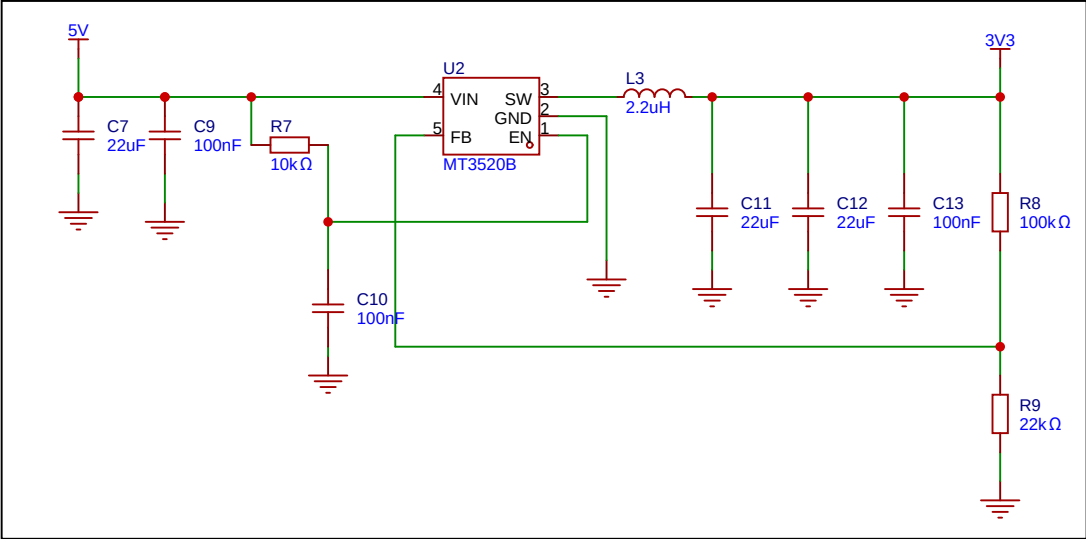
DCDC 5-3V3
