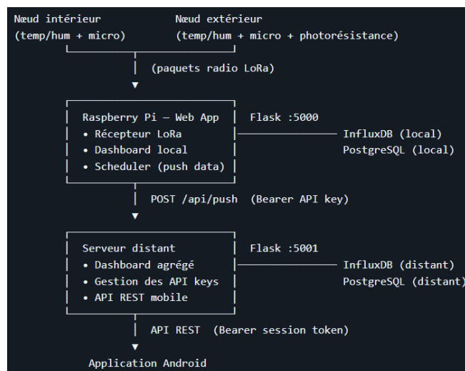
Figure 1 - Architecture réseau et flux de données de l'écosystème Beetter
