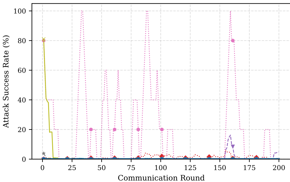
MNIST — Min-Max ASR (f=20)
