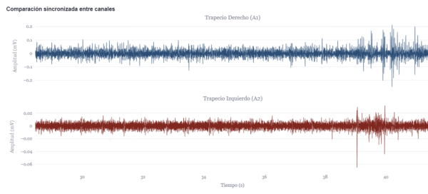
Fig. 4. Comparación bilateral de la señal con mochila de una asa (PRIV2).
