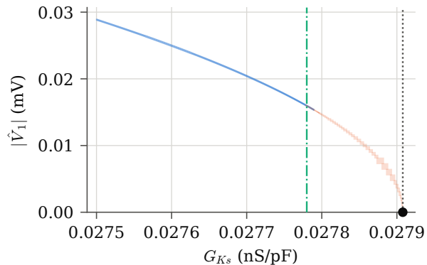
(d) detail of (b) at the Hopf point
