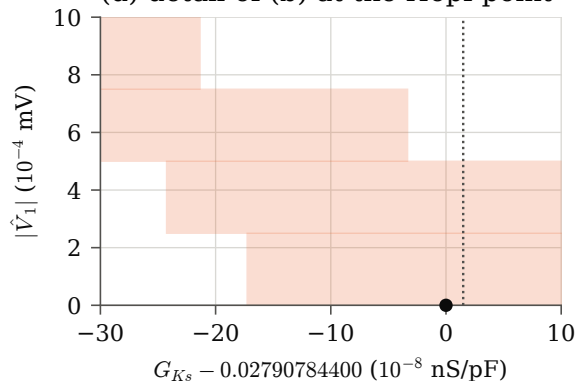
(d) detail of (b) at the Hopf point
