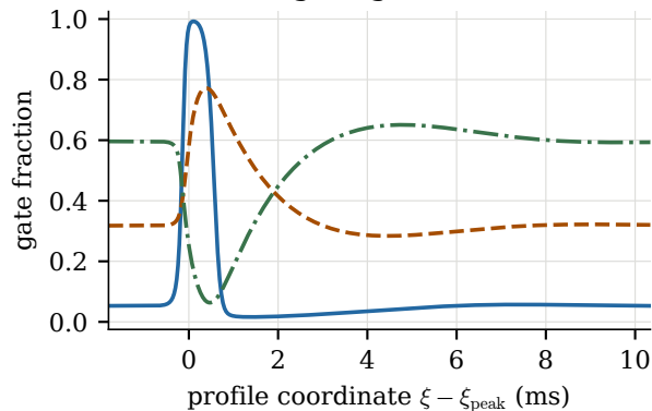
(d) 6.3 °C: gating variables
