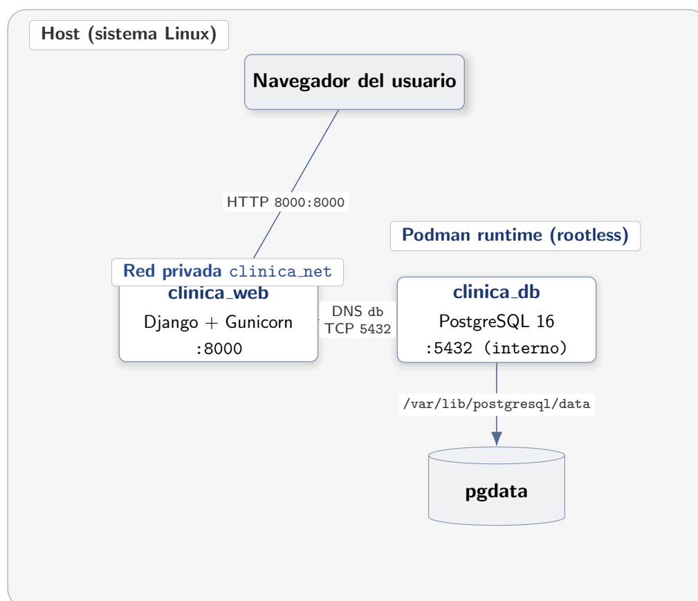
Figura 8: Arquitectura de contenedores del sistema.
