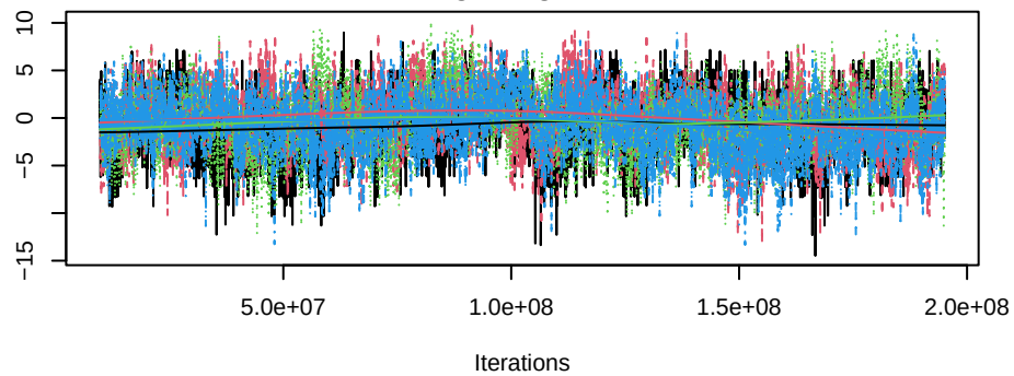
Trace of gwesp.OTP.fixed.0.025
