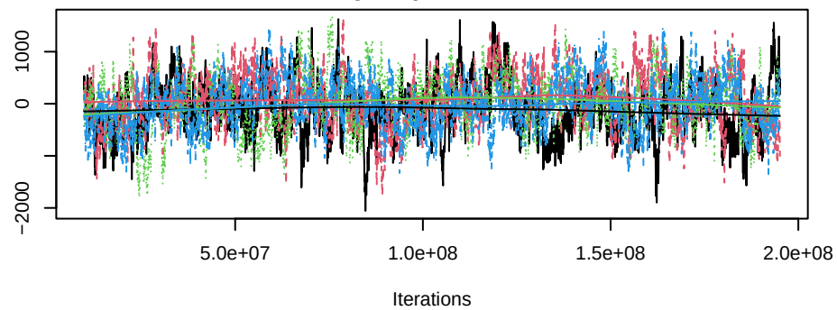
Trace of gwdsp.OTP.fixed.0.025
