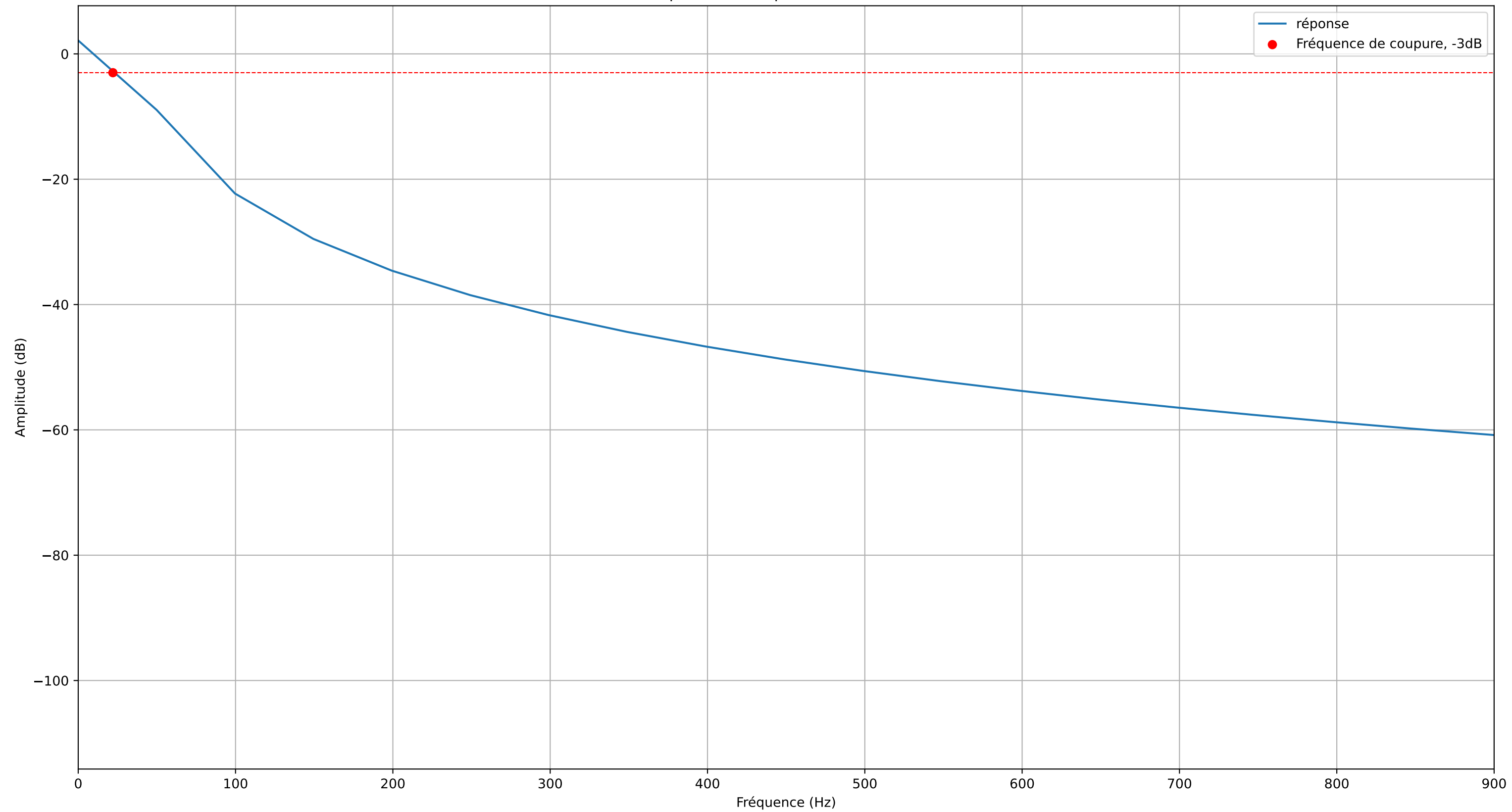
Réponse en fréquence du filtre RIF
