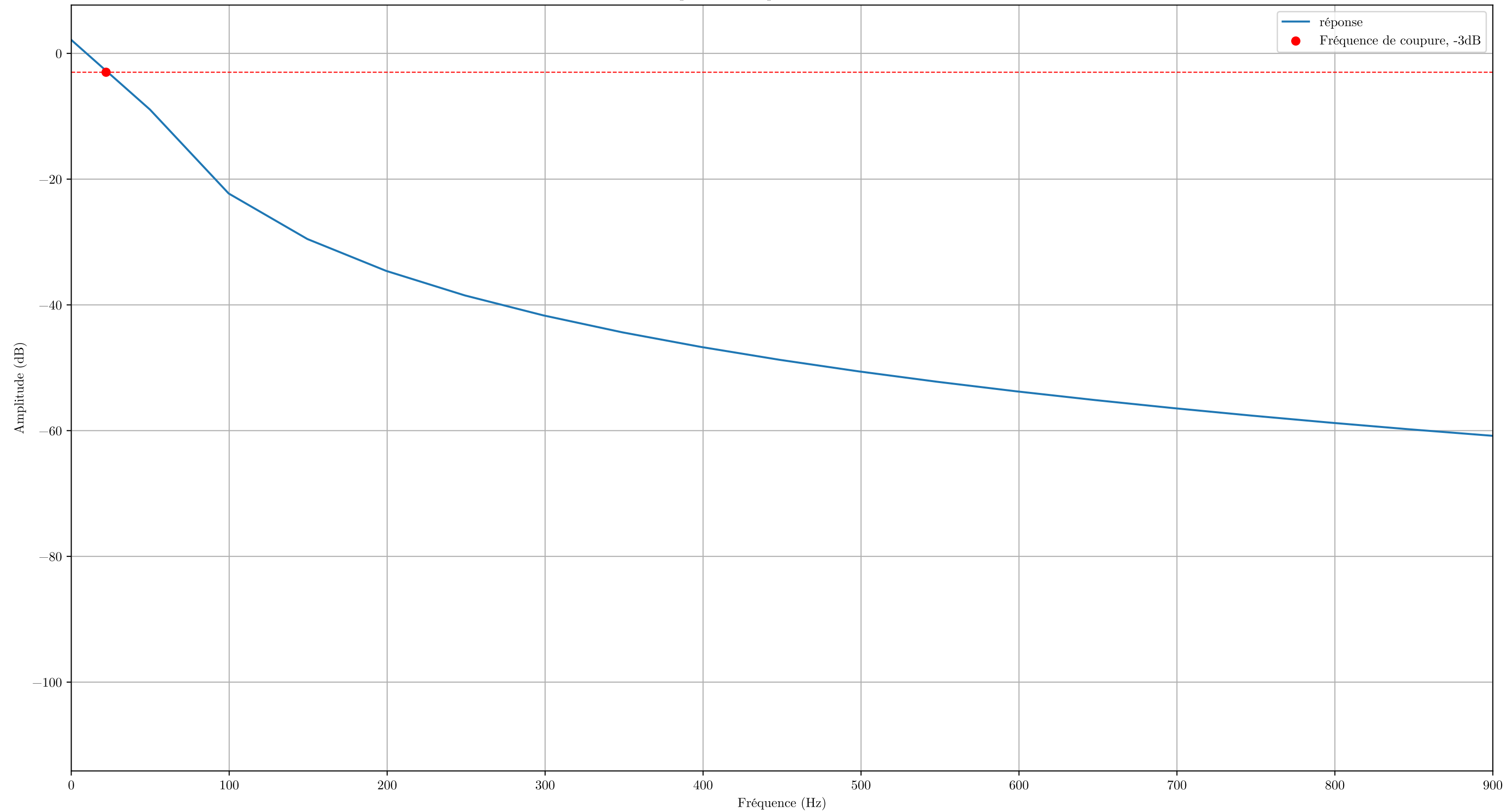
Réponse en fréquence du filtre RIF
