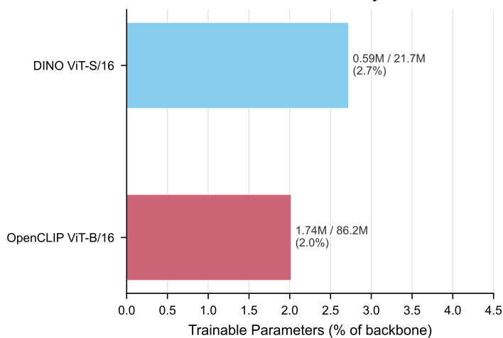
Parameter Efficiency
