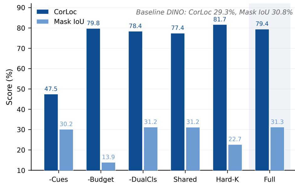
(d) Component Ablation (DINO, VOC)
