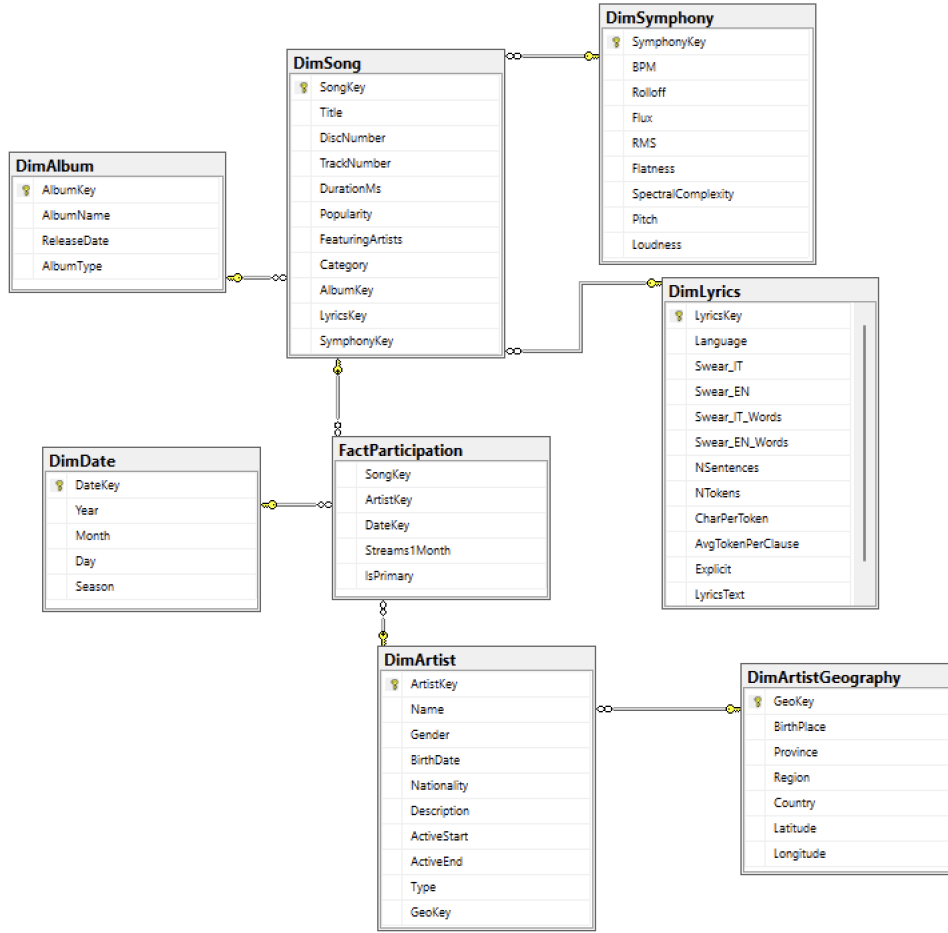
Figure 2: Schema concettuale
