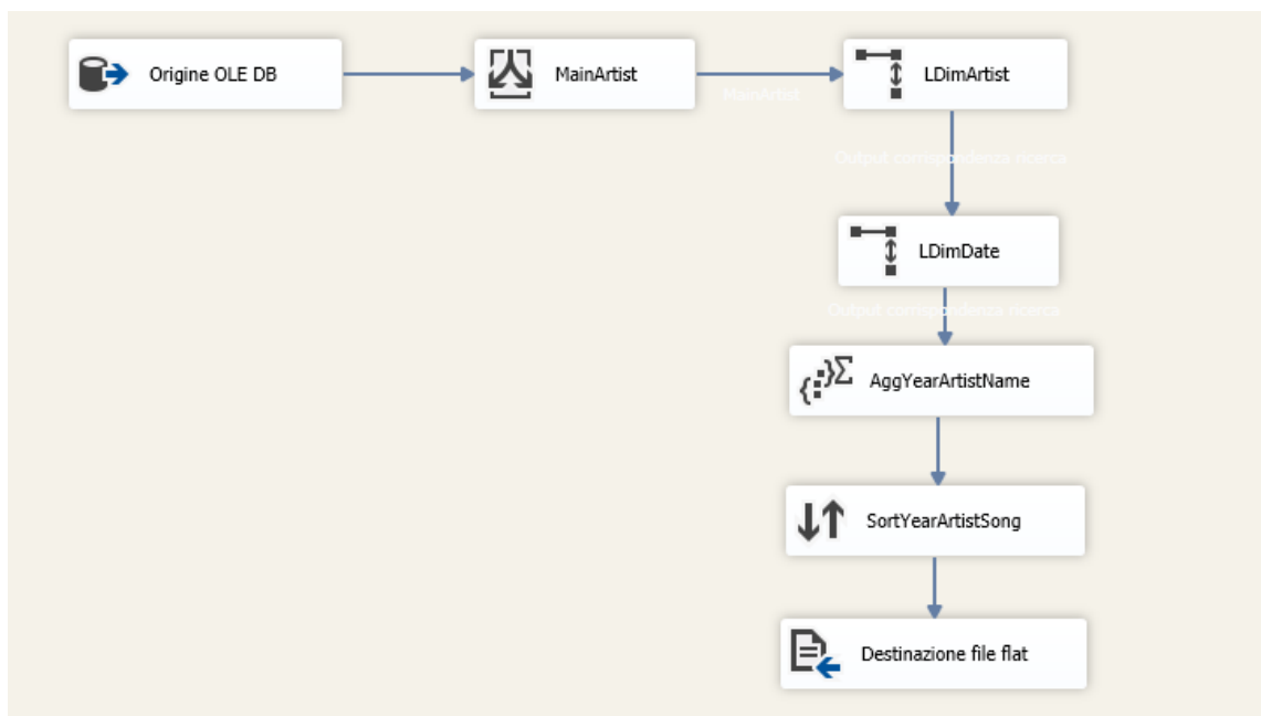
Figure 2: Data Flow SSIS per il calcolo del numero di canzoni pubblicate per artista e anno
