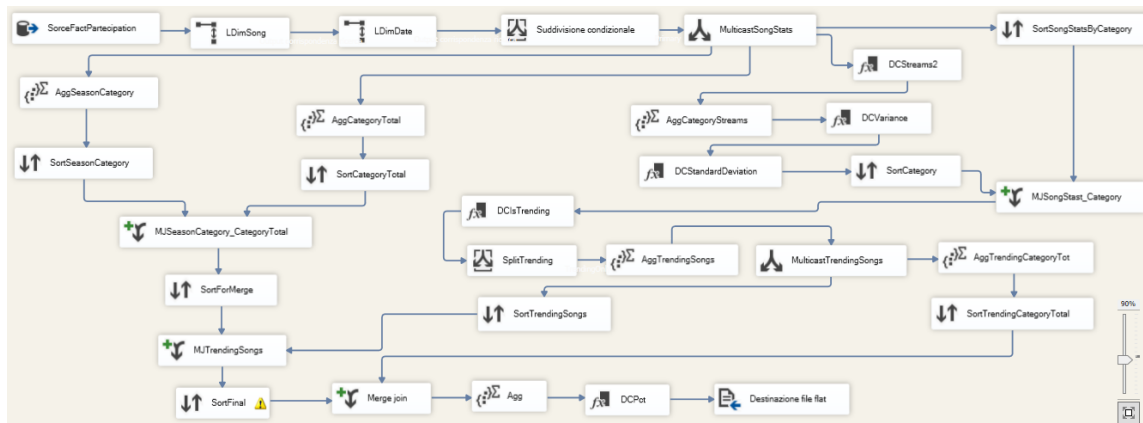
Figure 6: Data Flow SSIS per l'analisi delle canzoni trending per stagione e categoria
