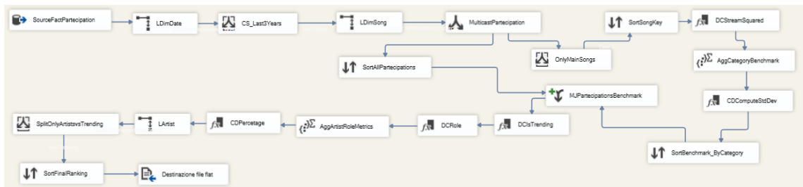
Figure 7: Data Flow SSIS per l'analisi delle performance degli artisti come primary e featured
