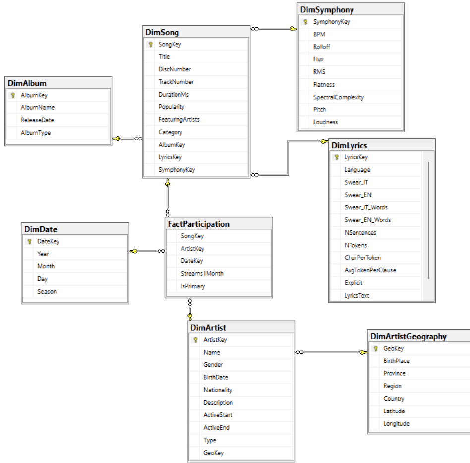
Figure 2: Schema concettuale
