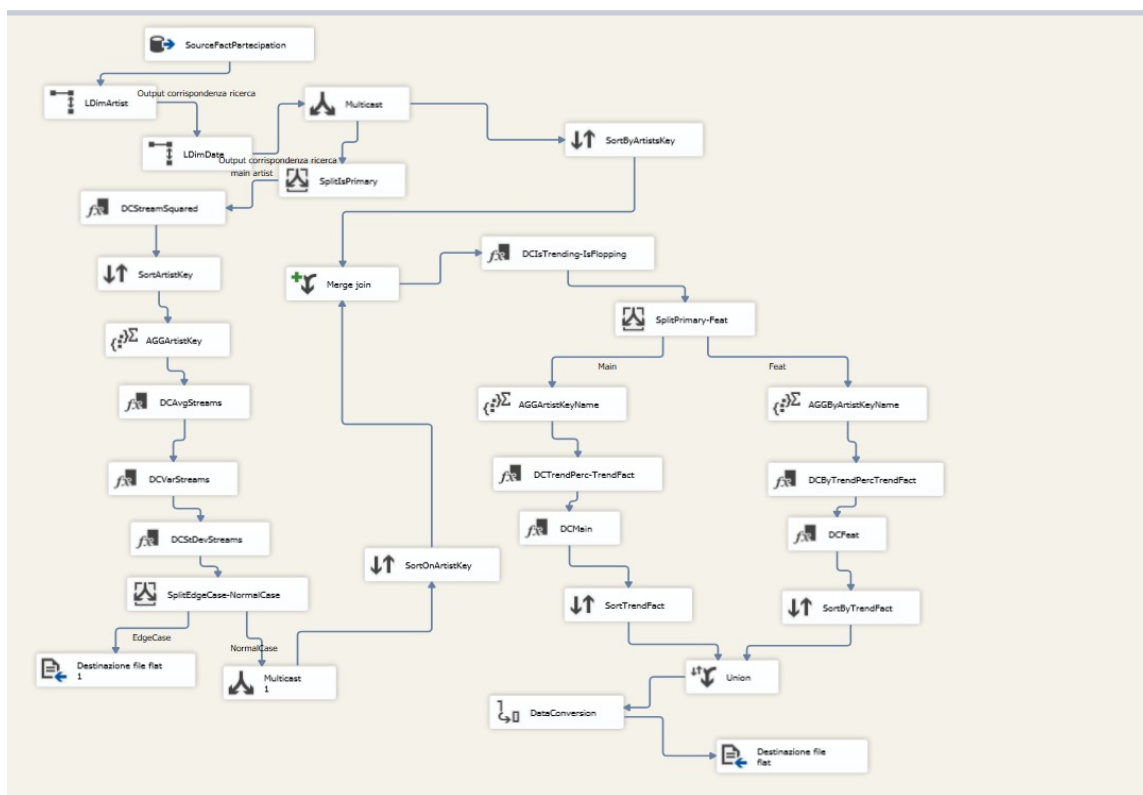
Figure 7: Data Flow SSIS per il calcolo degli indicatori di Trending per artista
