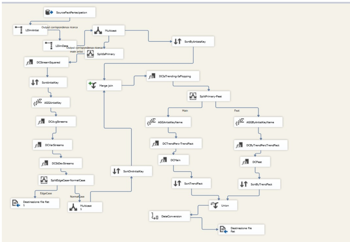
Figure 4: Data Flow SSIS per il calcolo degli indicatori di Trending per artista
