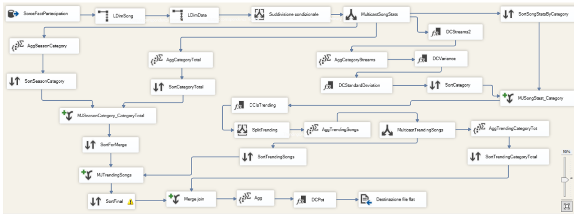
Figure 5: Data Flow SSIS per l'analisi delle canzoni trending per stagione e categoria
