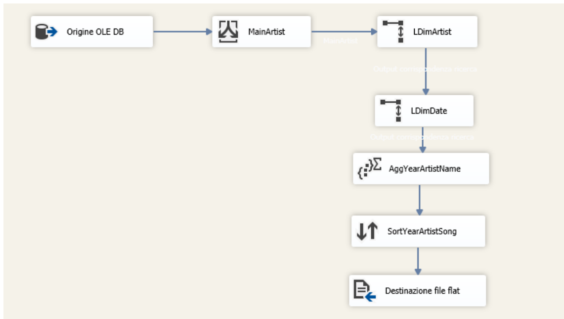
Figure 1: Data Flow SSIS per il calcolo del numero di canzoni pubblicate per artista e anno
