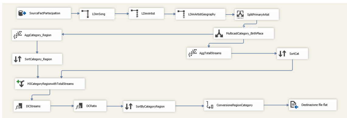
Figure 3: Data Flow SSIS per il calcolo del rapporto di stream per categoria e regione
