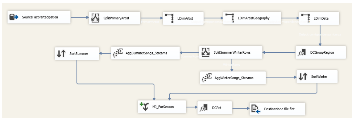
Figure 2: Data Flow SSIS per il calcolo del Summer–Winter Score per regione
