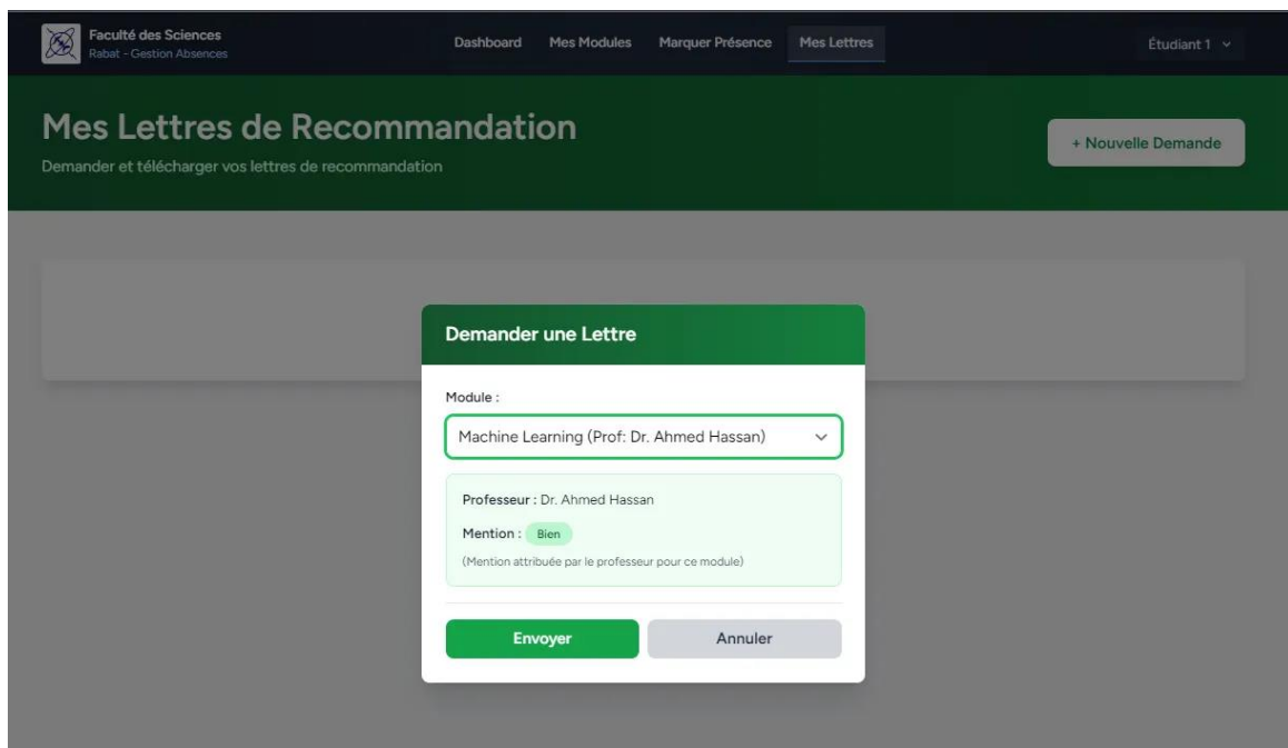
Figure 30 : Screenshot de la section « Meslettres» pour demander une lettre de recommandation
