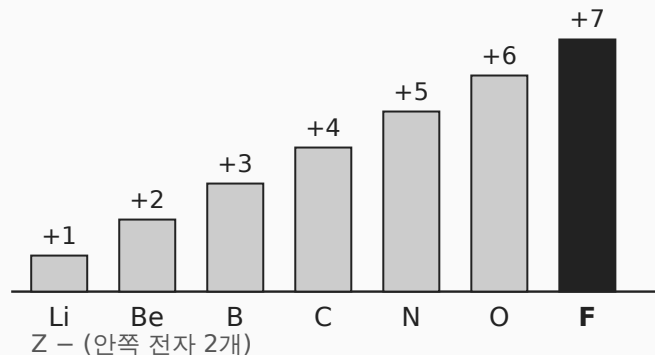
2주기 원자가 전자가 느끼는 핵전하(어림)
