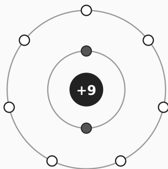
F : 안쪽 2개 · 바깥 7개
