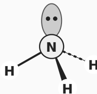
NH 3 · 삼각뿔형 비공유 1 · 107°
