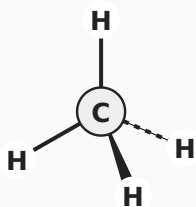
CH 4 · 정사면체 비공유 0 · 109.5°
