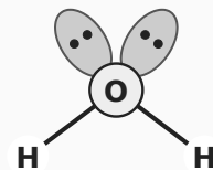
H 2 O · 굽은형 비공유 2 · 104.5°
