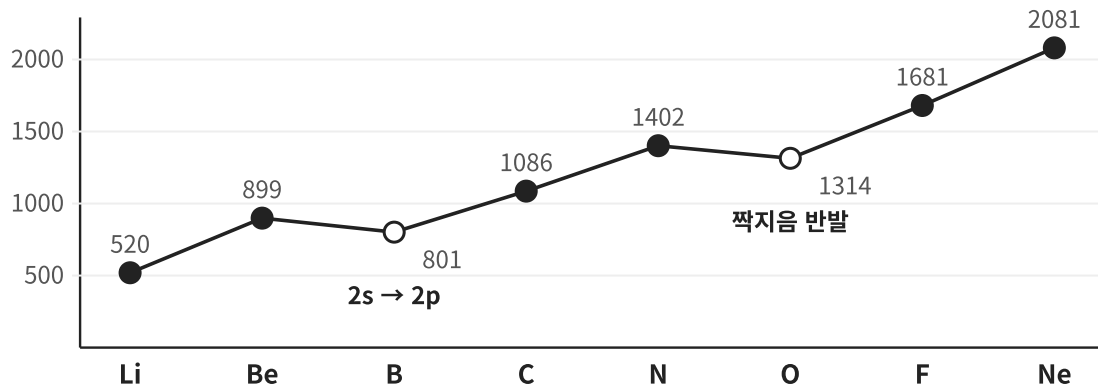
제1 이온화 에너지(kJ/mol) · 흰 점이 꺾인 자리
