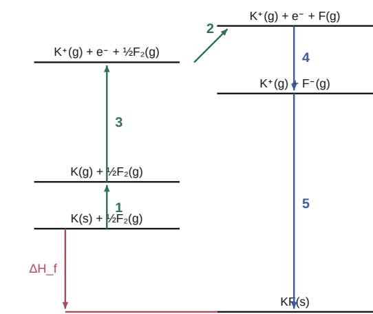
KF Born-Harber 순환 · 단계 1-5 · 재작도 — 원본 그림의 내용을 글 서술에서 다시 그린 것입니다
