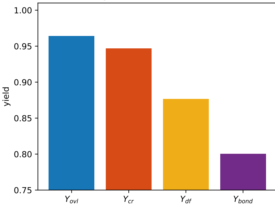
Fig. 17: W2W Full, 0.3 um
