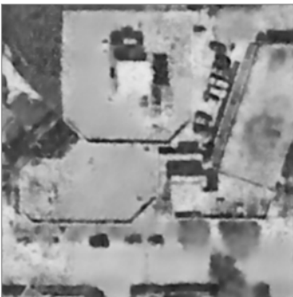
(e) SAR-CAM
