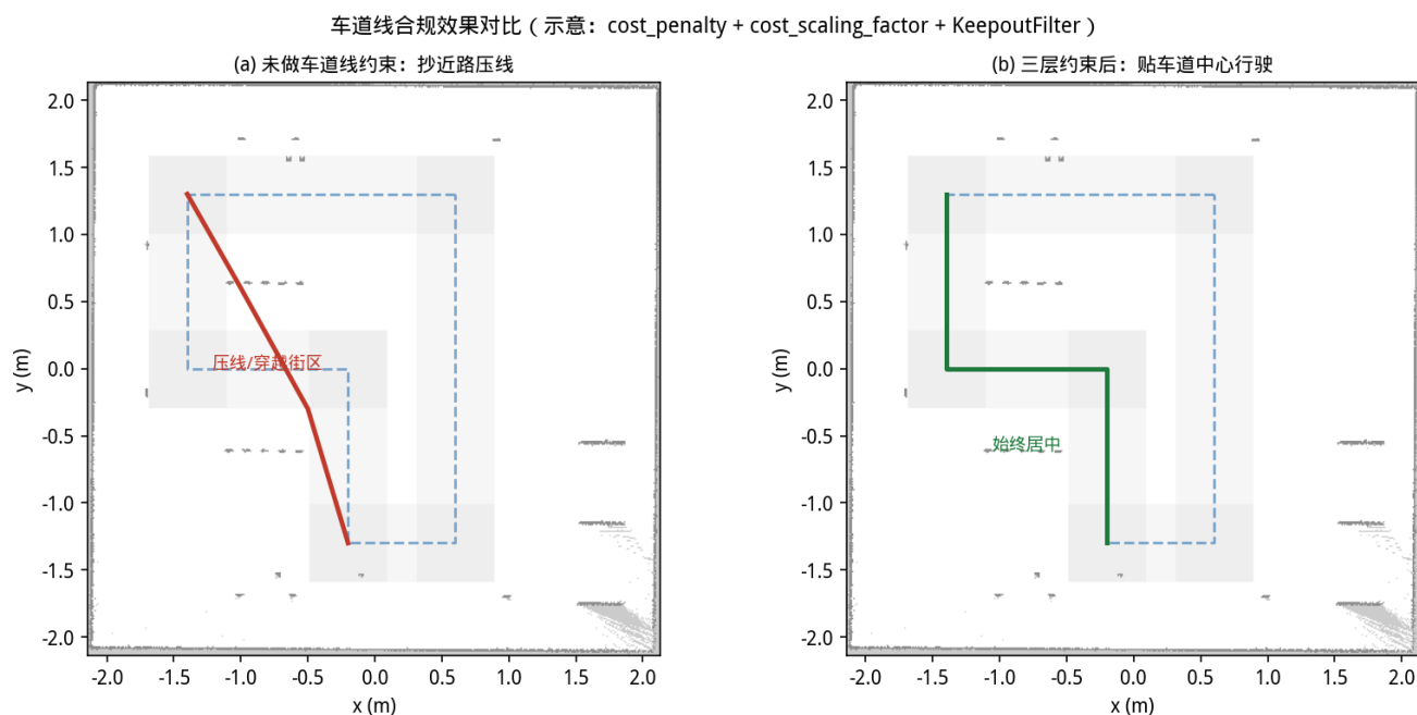
图 6 为示意：左图展示无车道线约束时规划器会抄近路穿过街区、压越车道线；右图展示 cost_penalty + cost_scaling_factor + KeepoutFilter 三层约束生效后 全局路径始终贴车道中心线行驶。真实 RViz 对比可在加载 KeepoutFilter 前后各截一张。
