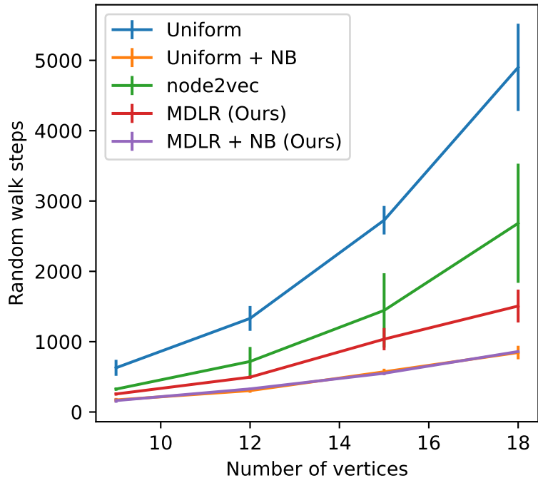
Edge cover time C_E(G)
