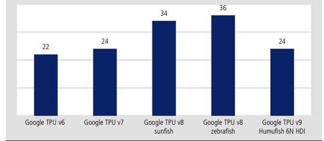
圖 2：TPU V9 PCB 走高層數與多層 HDI
