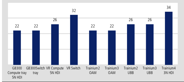
圖 1：AWS T4 走高層數與多層 HDI
