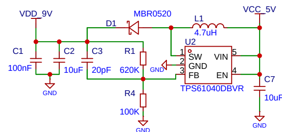
升压电路5V转9V
