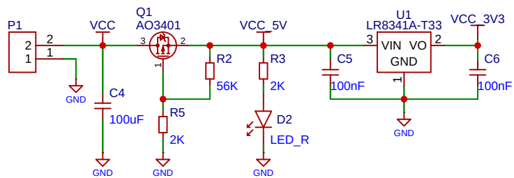
电源输入保护
