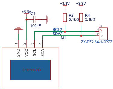
128x64 OLED显示器
