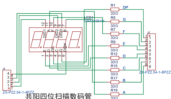
共阳四位扫描数码管
