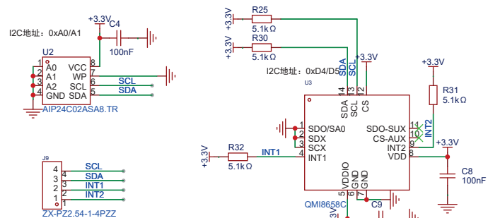
I2C总线上的EEPROM+六轴IMU
