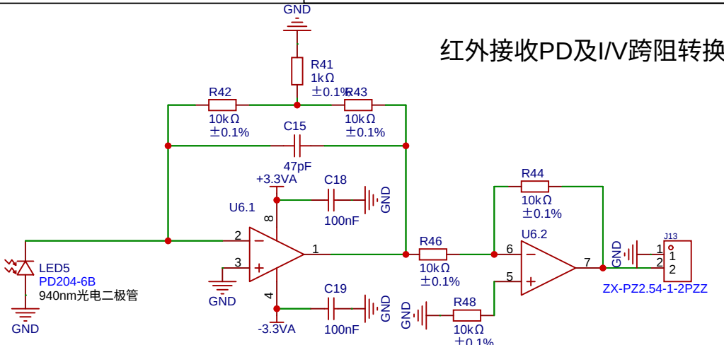
底板
