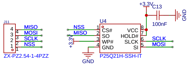
SPI总线上的FLASH
