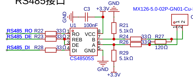
RS485接口
