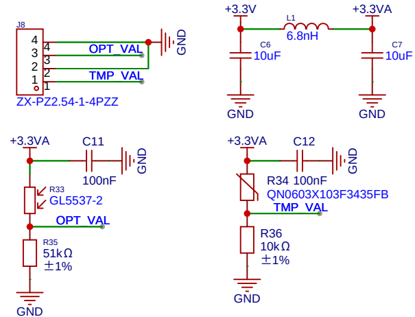
光敏/温敏传感器
