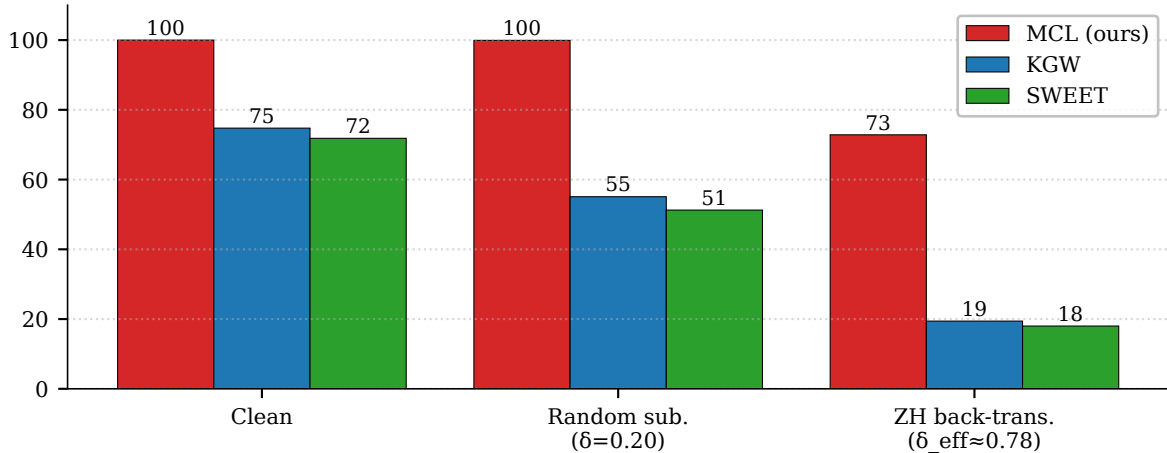
TPR @ FPR=0.01 (%)
