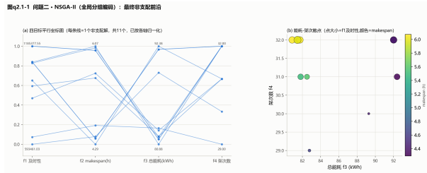
(a) NSGA-II 四目标 Pareto 前沿
