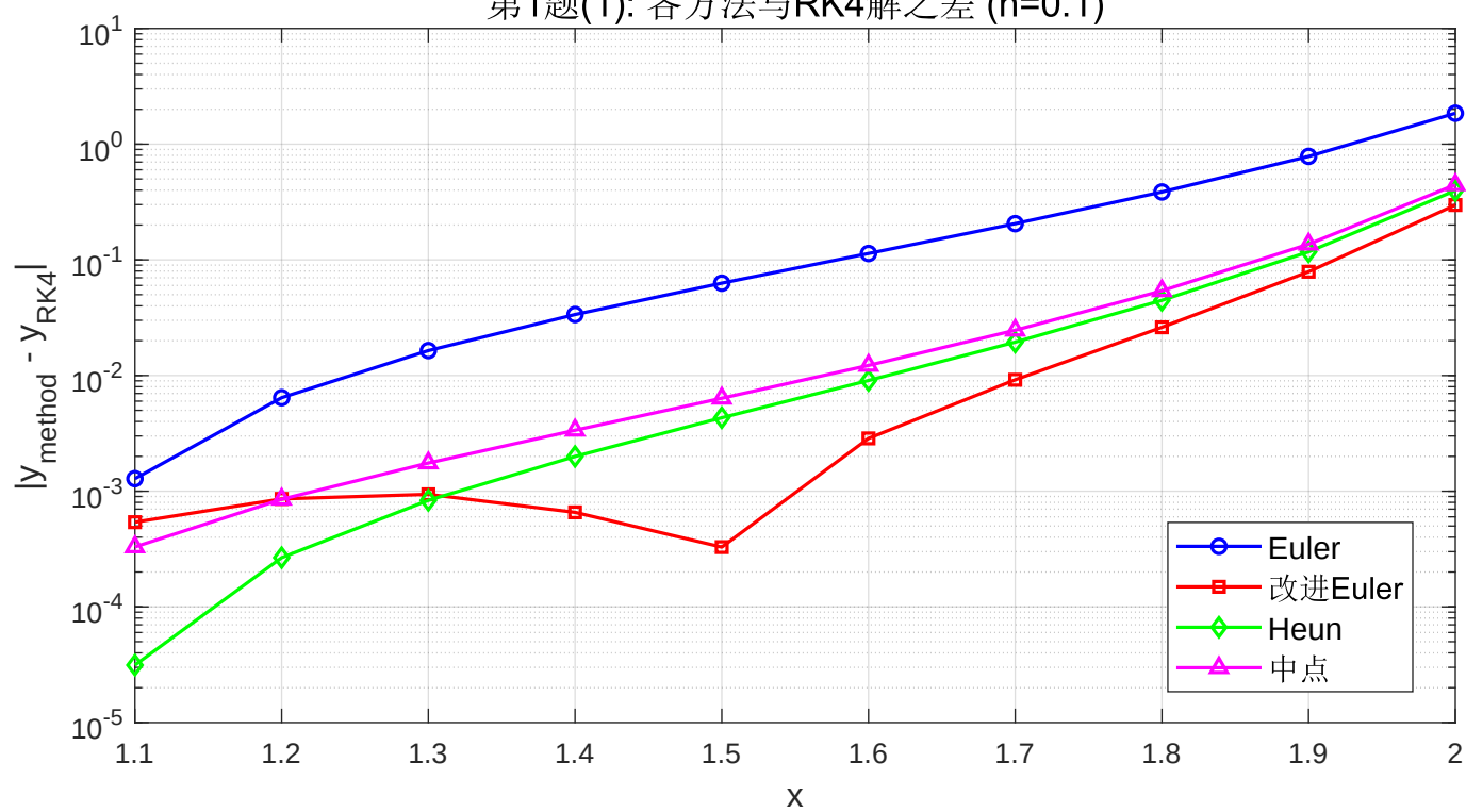
第1题(1): 各方法与RK4解之差 (h=0.1)
