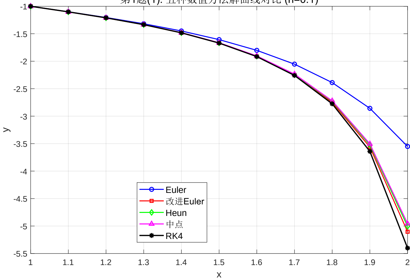
第1题(1): 五种数值方法解曲线对比 (h=0.1)
