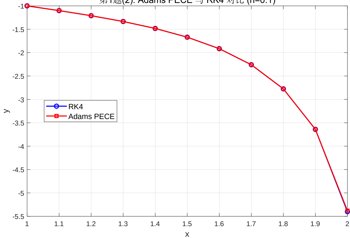
第1题(2): Adams PECE 与 RK4 对比 (h=0.1)
