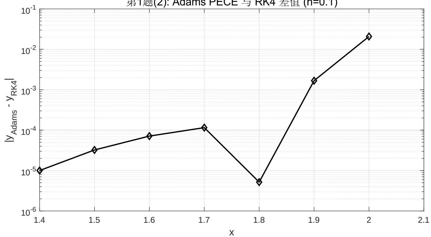
第1题(2): Adams PECE 与 RK4 差值 (h=0.1)
