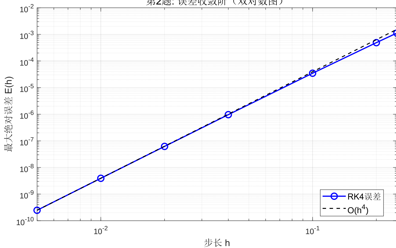
第2题: 误差收敛阶 (双对数图)
