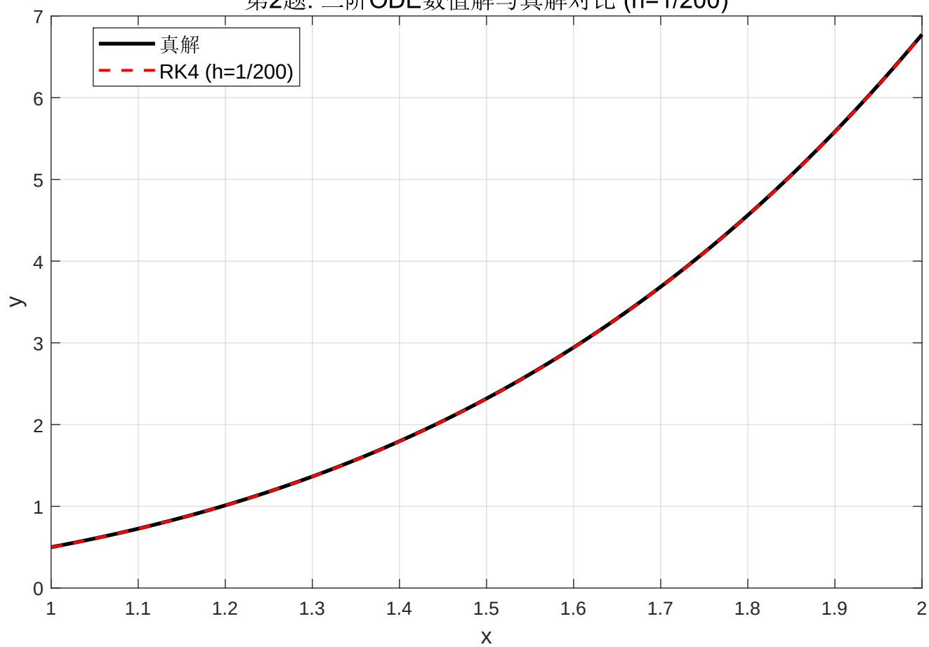
第2题: 二阶ODE数值解与真解对比 (h=1/200)
