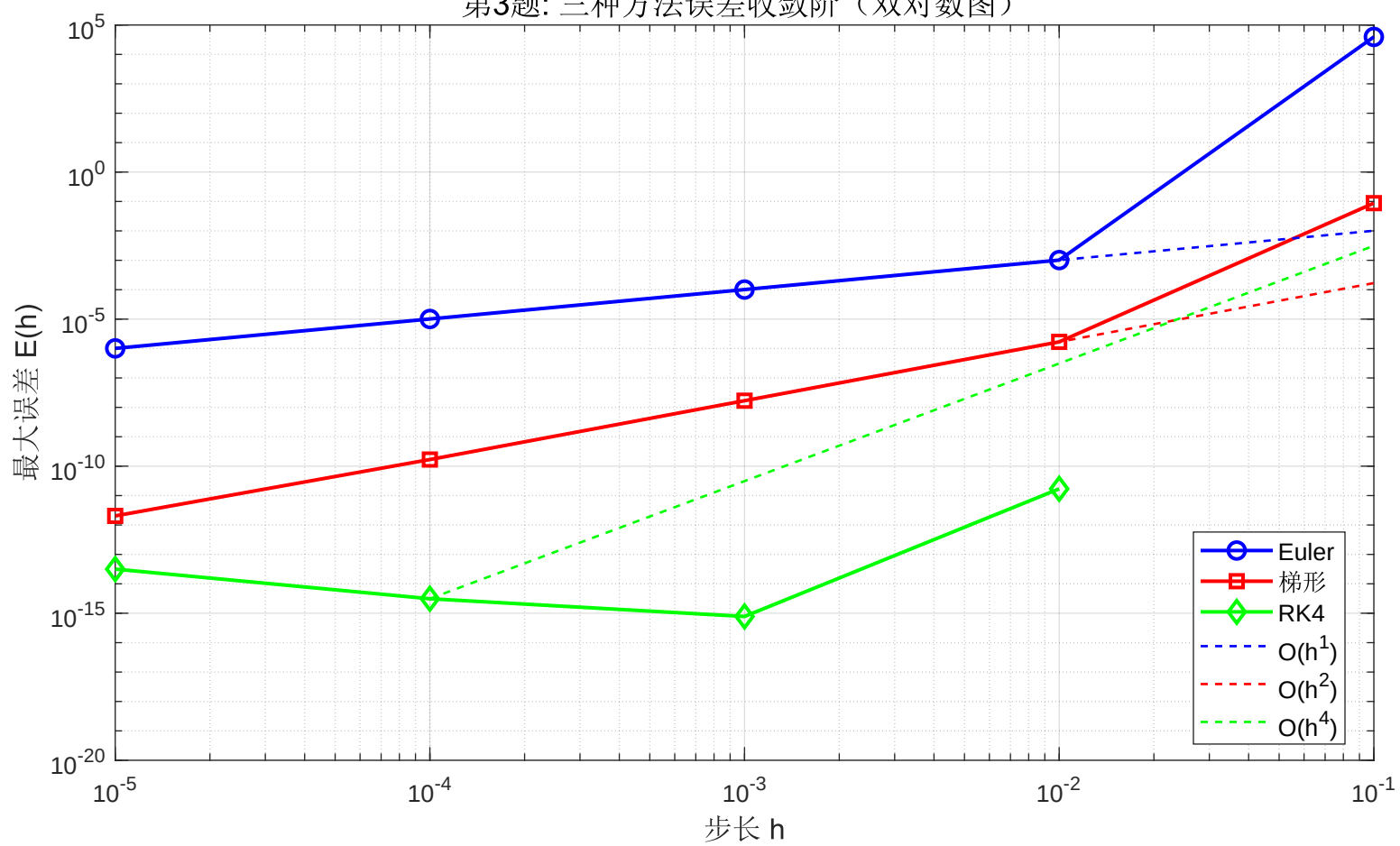
第3题: 三种方法误差收敛阶 (双对数图)
