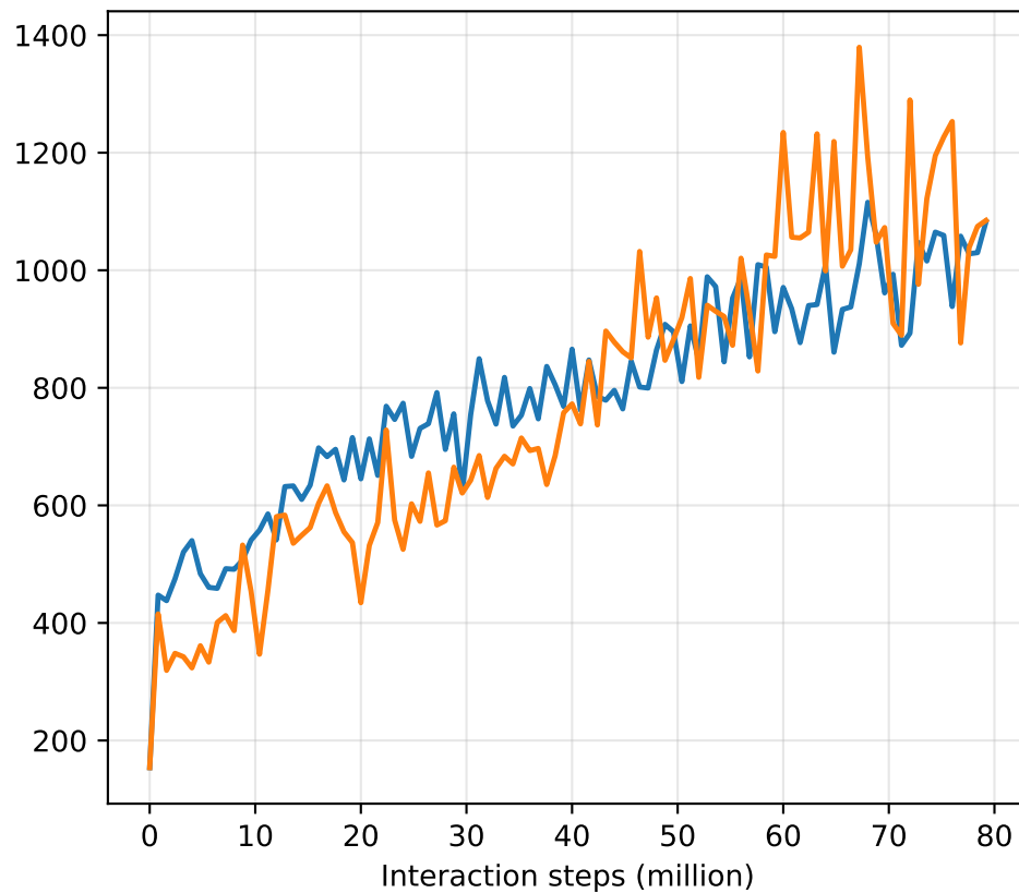
Humanoid-v5
