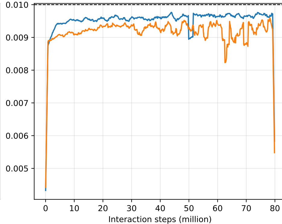
Humanoid-v5
