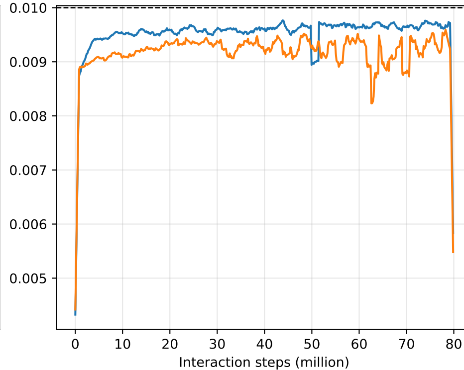
Humanoid-v5
