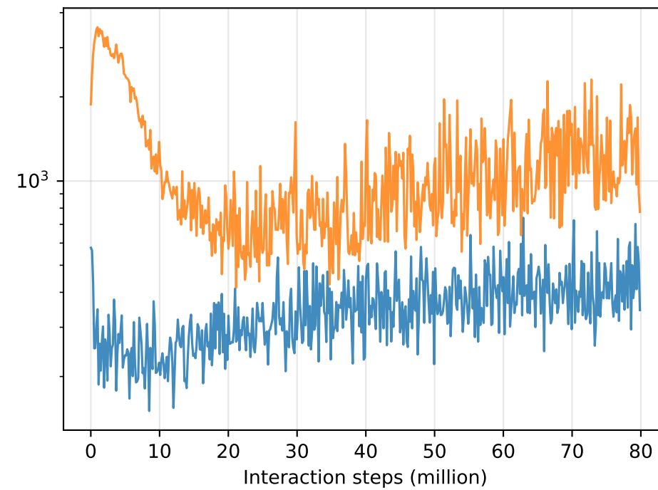
Humanoid-v5
