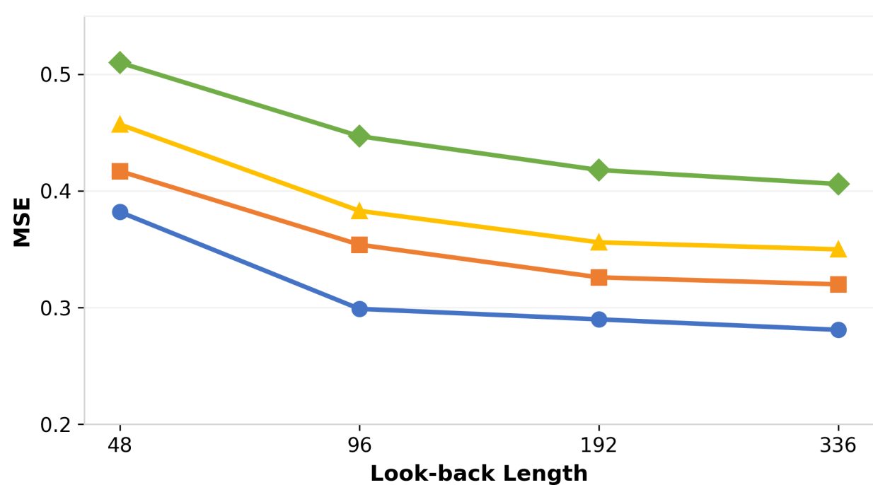
ETTm1
