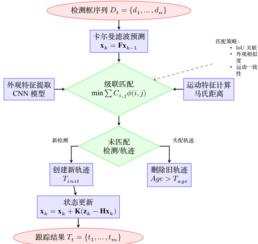
图 4-5: DeepSORT 算法框架
